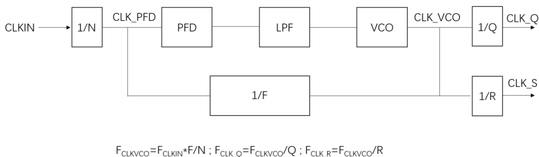
图5-65 锁相环系统
