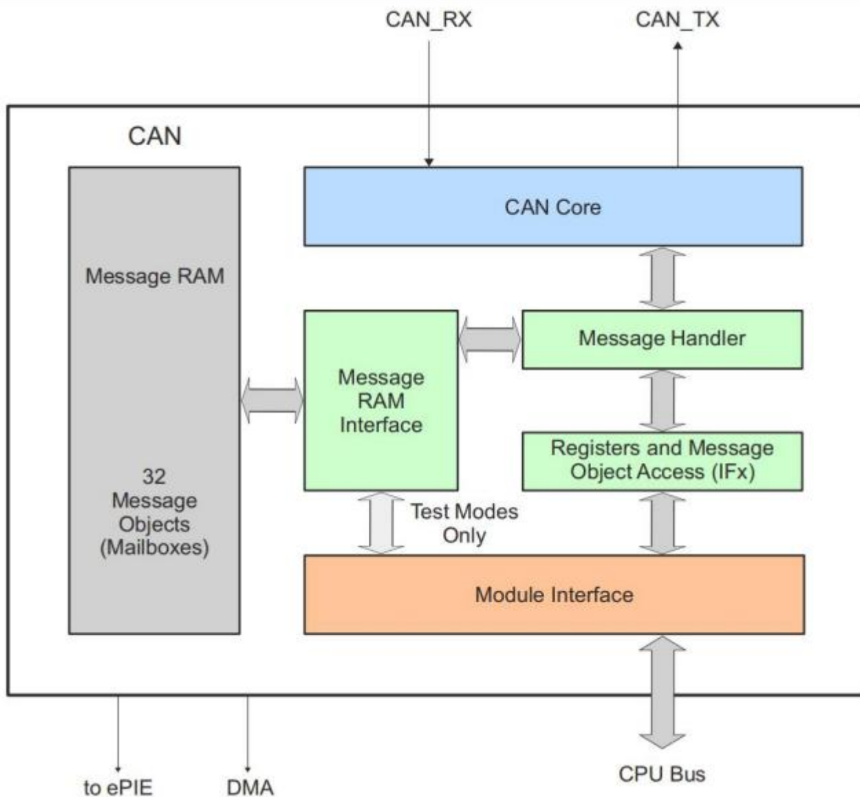
图 5- 46. CAN 框图
