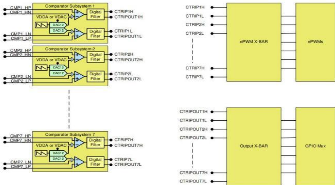
图 5-25 CMPSS 连接
