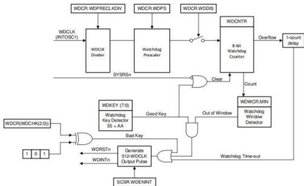
图 6-4. 看门狗
