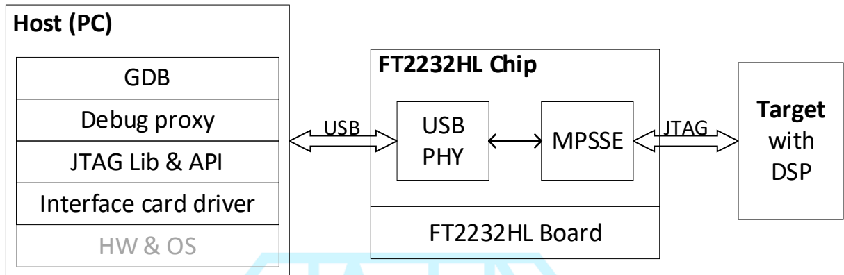
图 2：基本结构
