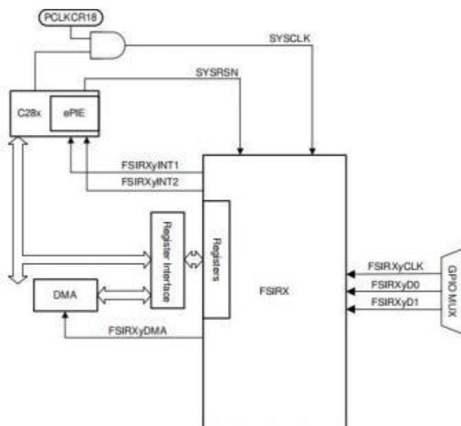
图 5-60. FSIRX CPU
