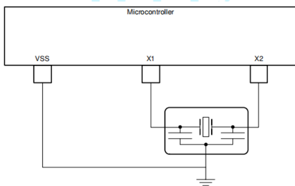
图5 - 68 外部谐振器
