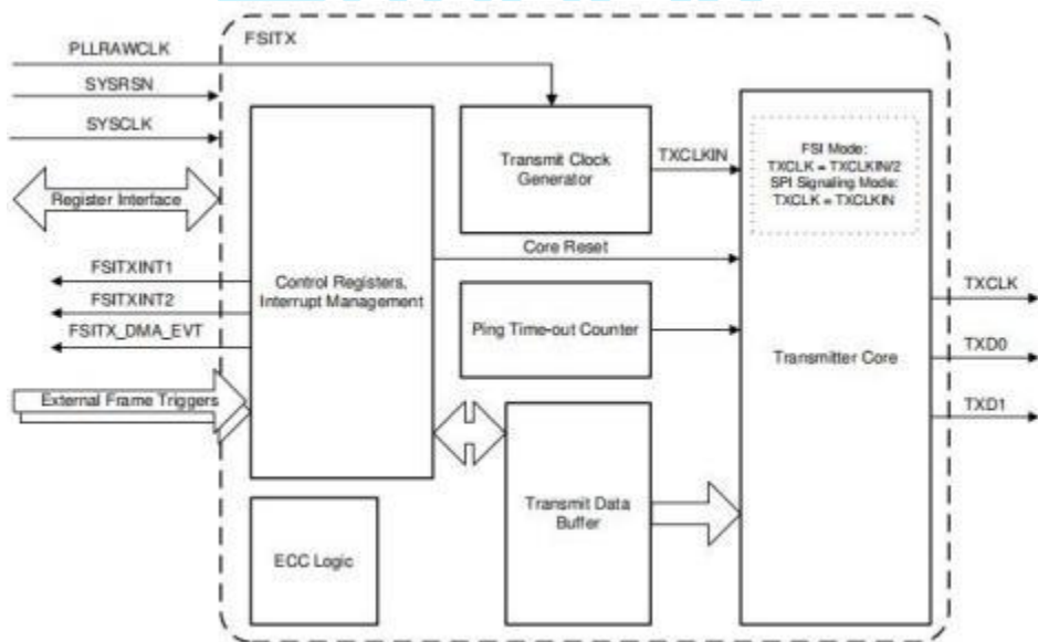
图 5-58. FSITX 框图
