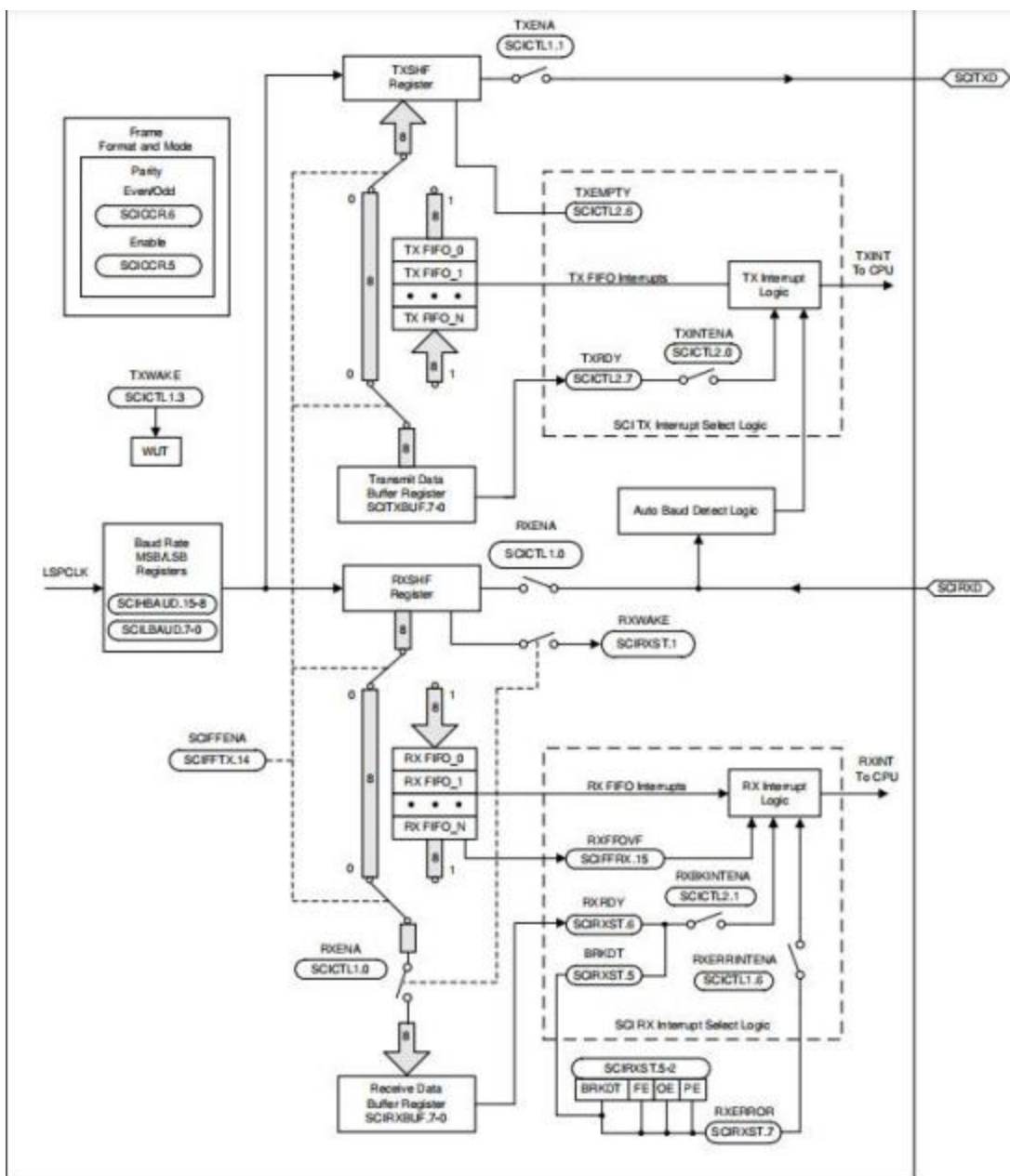
图 5-50. SCI 框图
