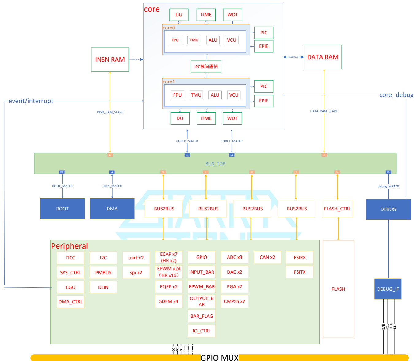
图 3-1 功能框图
