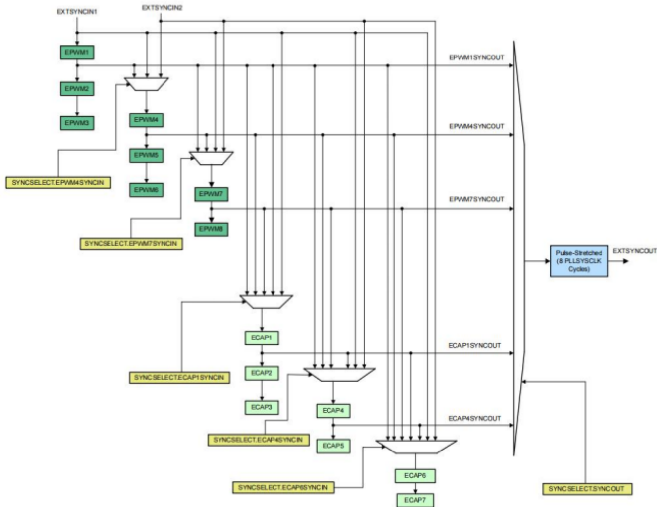
图 5-37. 同步链架构
