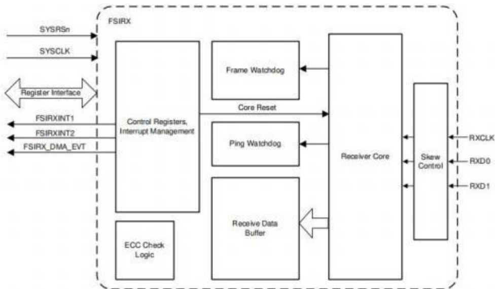
图 5-61. FSIRX 框图
