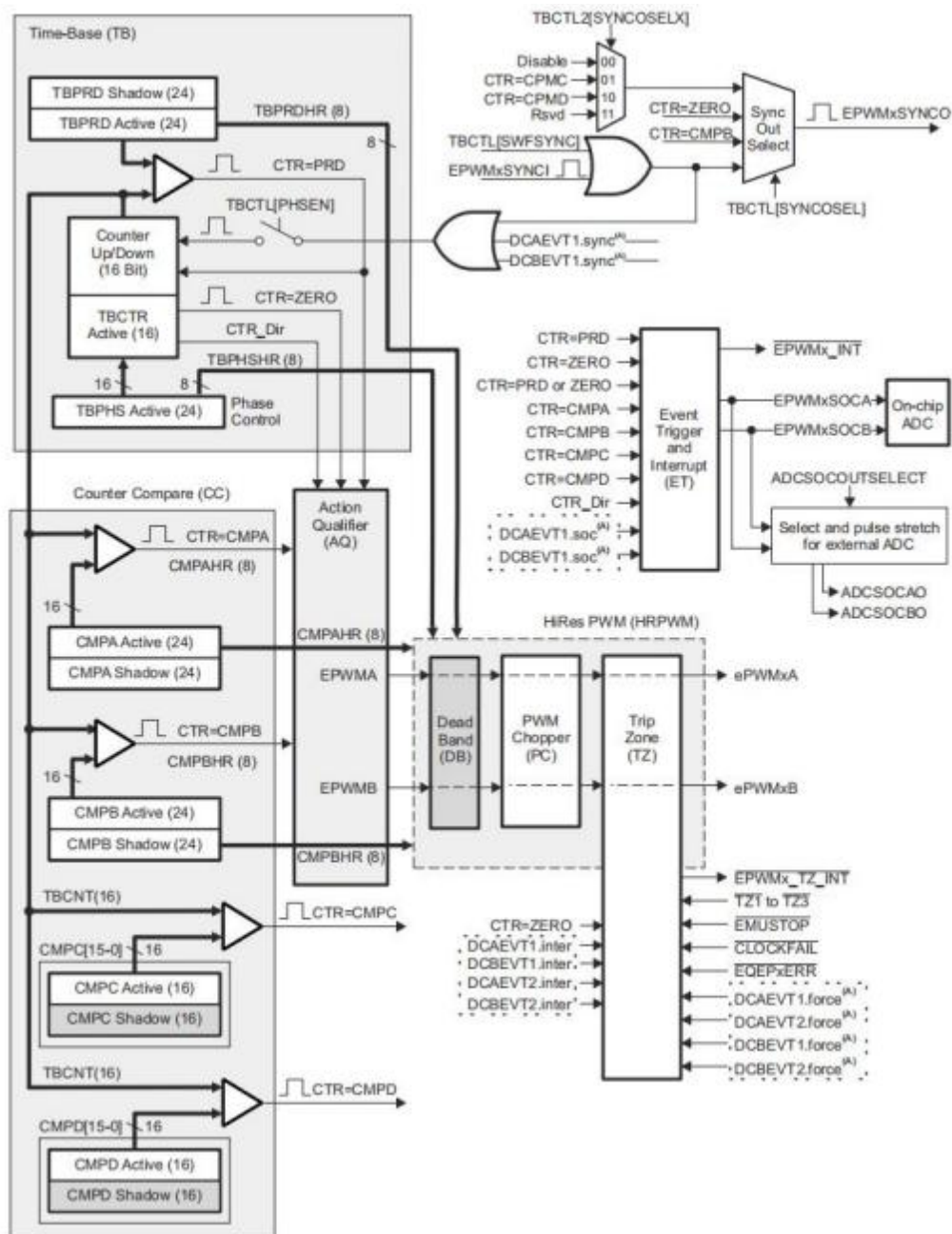
图 5-35. ePWM 子模块和关键内部信号连接
