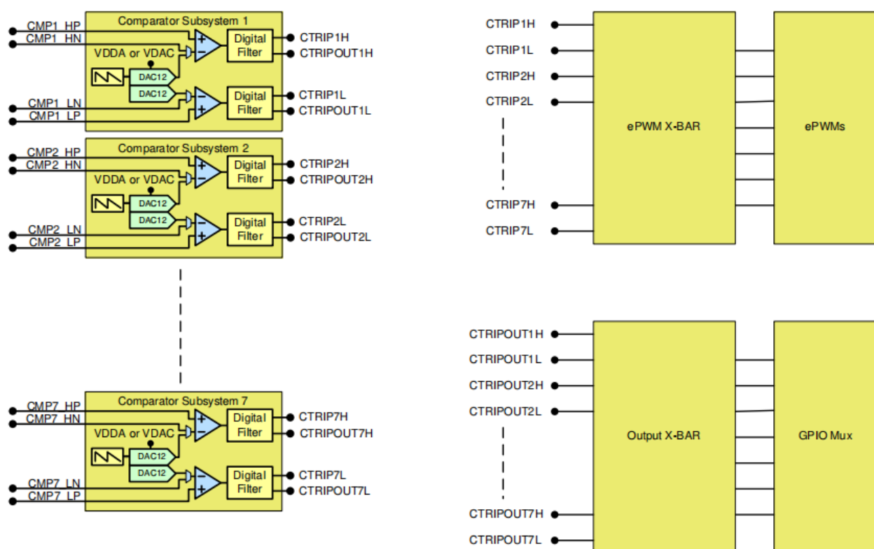
图 5-25 CMPSS 连接
