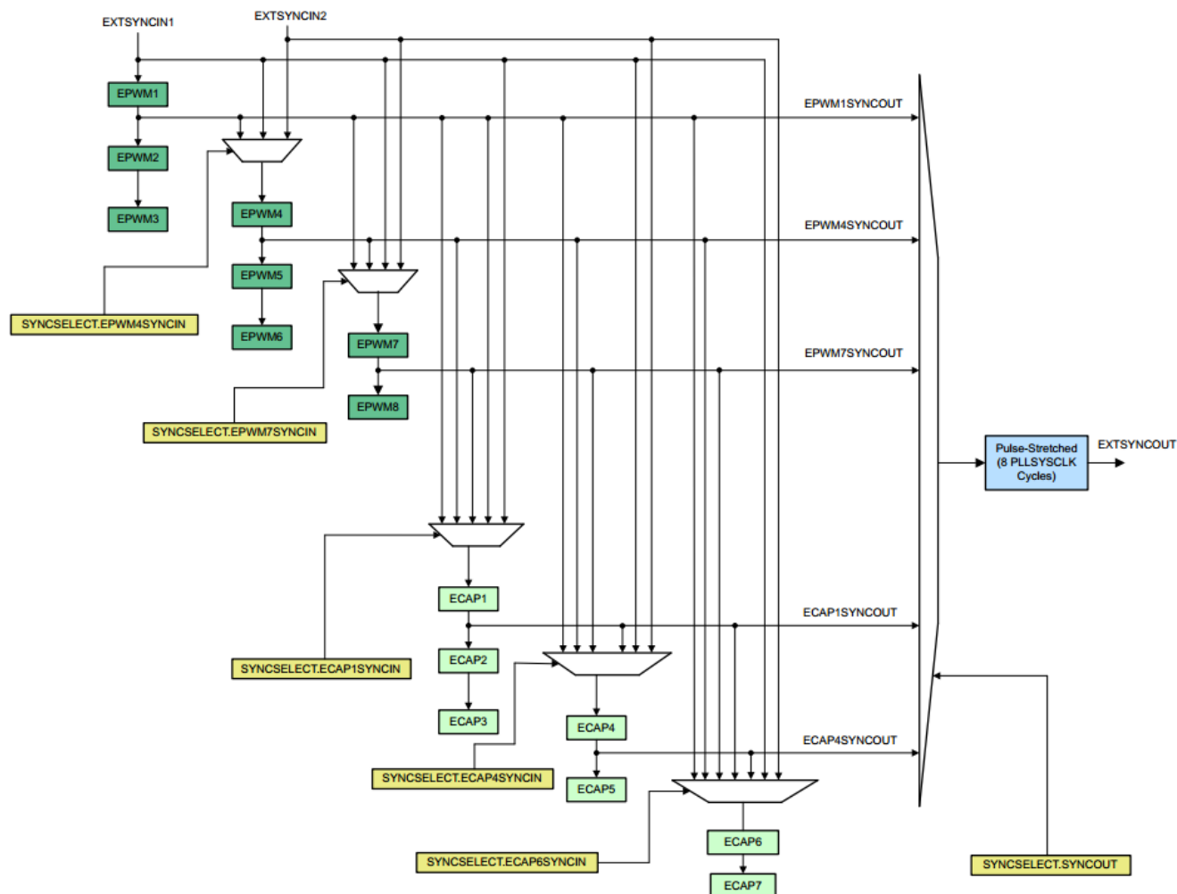
图 5-37. 同步链架构
