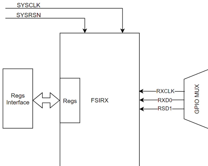
图 5-60. FSIRX CPU
