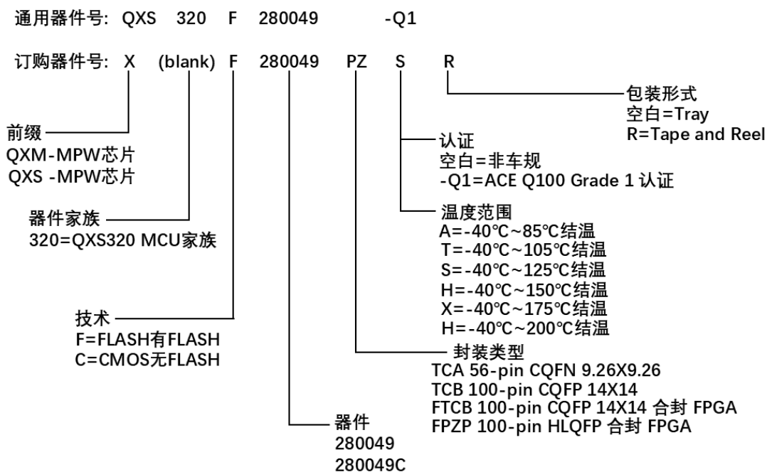
图 3-2 器件命名规则图
