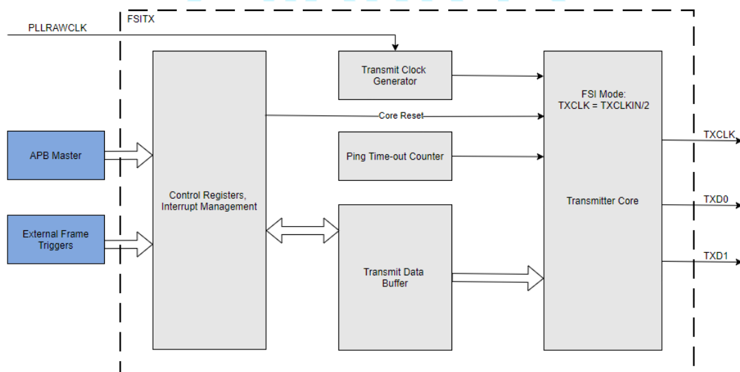
图 5-58. FSITX 框图
