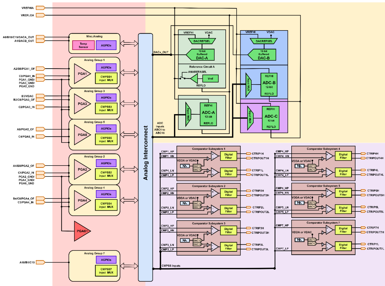
图 5-7 模拟子系统框图（64pin PM LQFP 封装）
