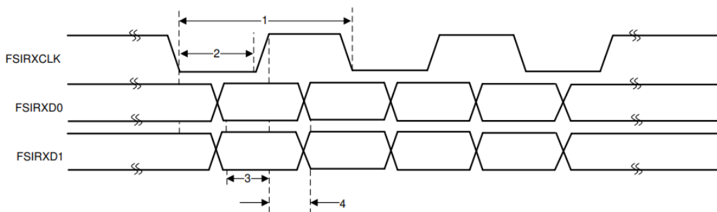
图 5- 62. FSIRX 时序
