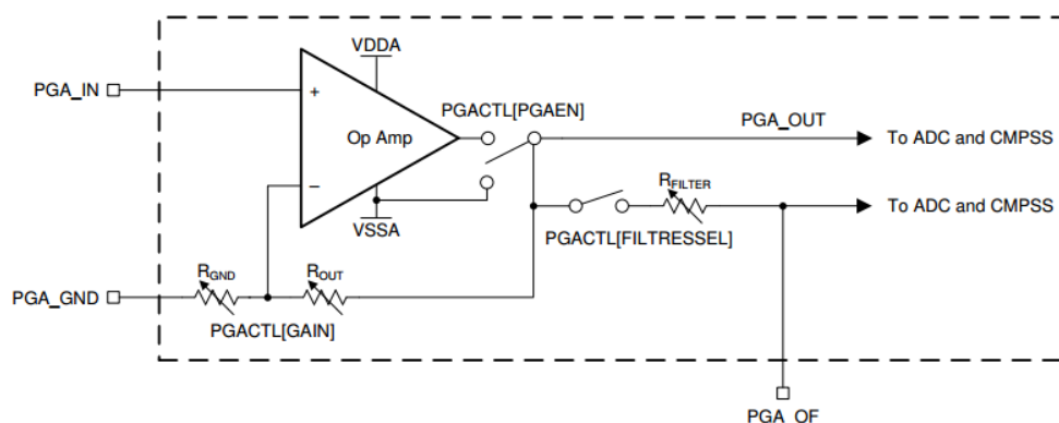
图 5-13. PGA 方框图
