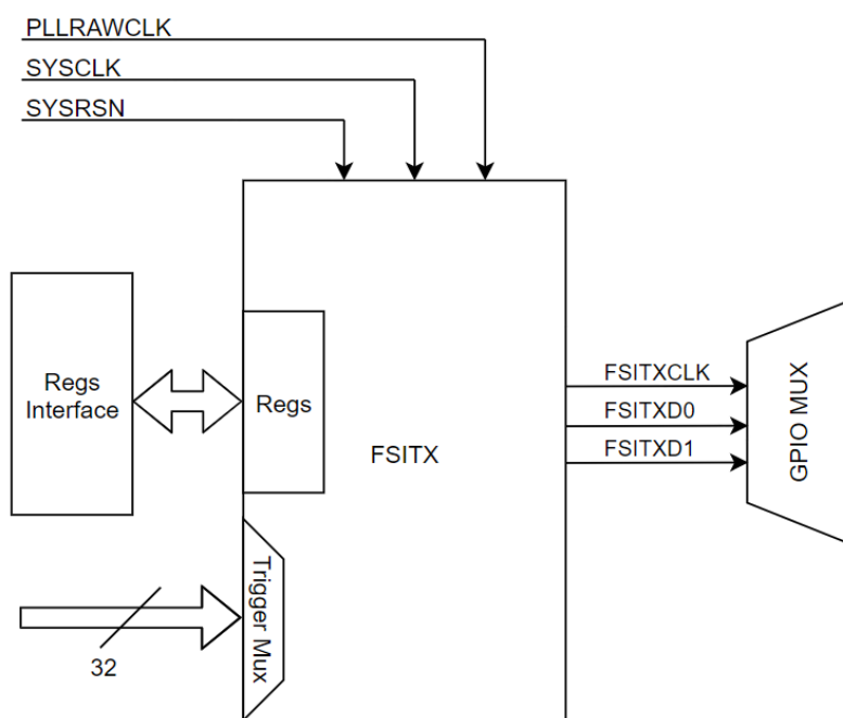
图 5-57. FSITX CPU 接口
