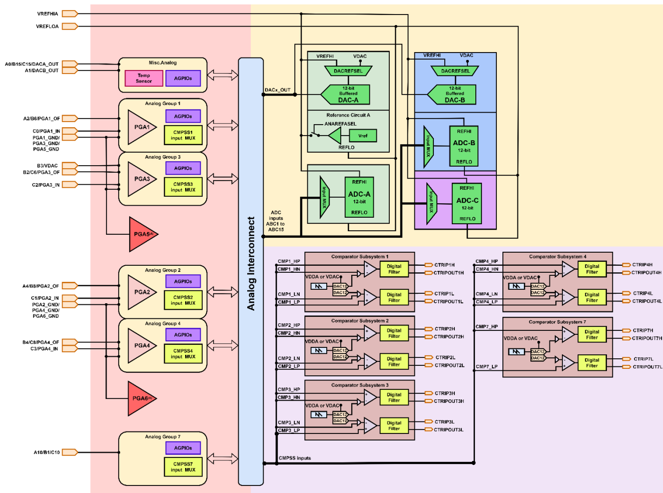
图 5-8 模拟子系统框图（56pin RSH VQFN 封装）
