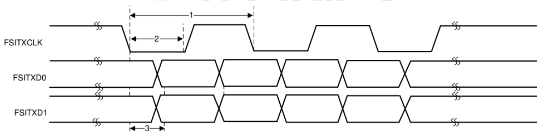
图 5- 59. FSITX 时序
