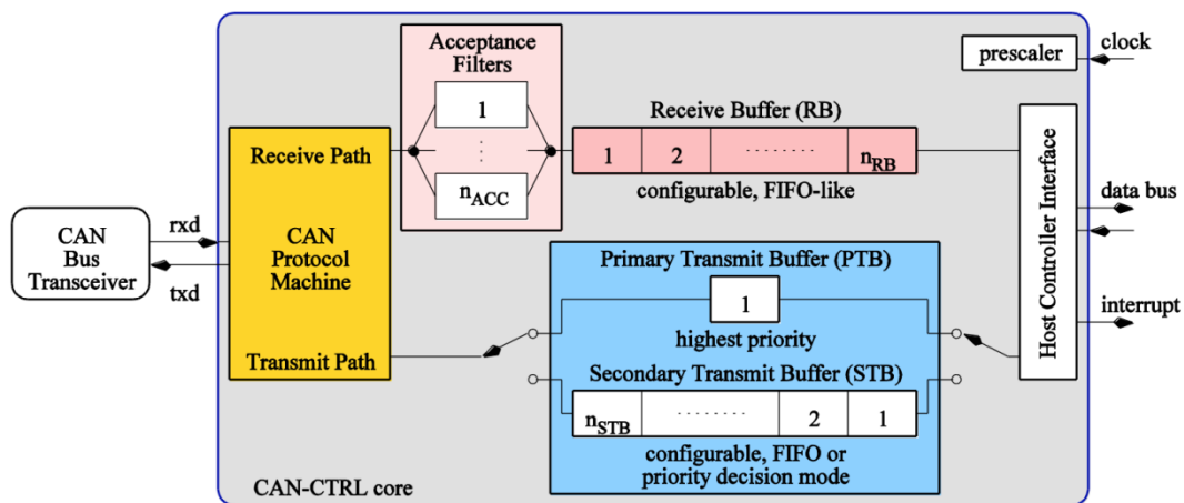
图 5- 46. CAN 框图
