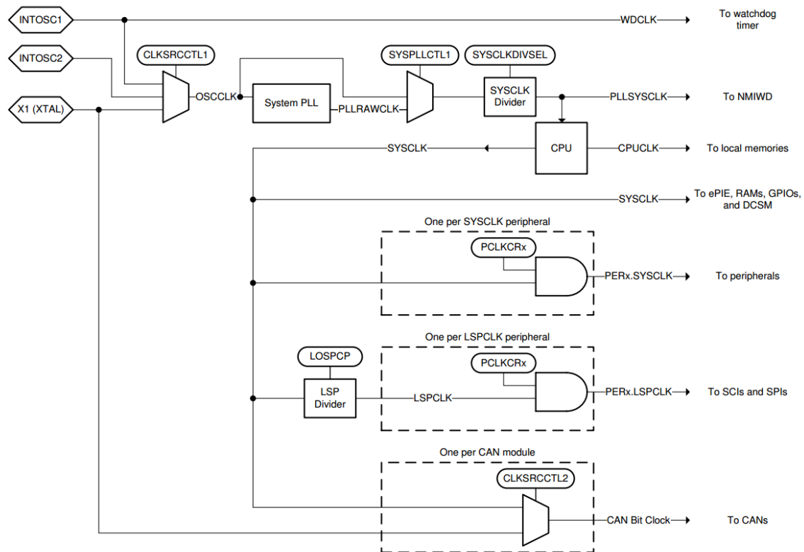
图5-64 系统时钟
