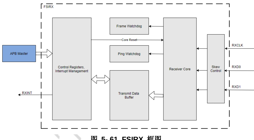
图 5-61. FSIRX 框图
